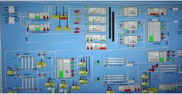
水资源综合利用项目水处理工艺流程图
